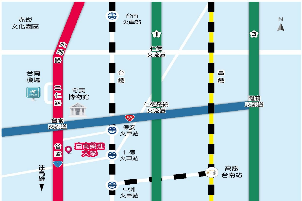
圖2、交通位置圖
